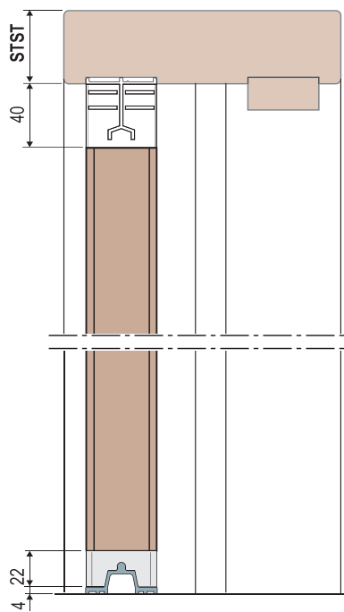
LISTEL N.1 WITH HIGH RAIL
