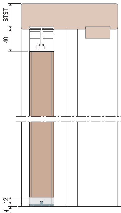
LISTEL N.1 WITH LOW RAIL
